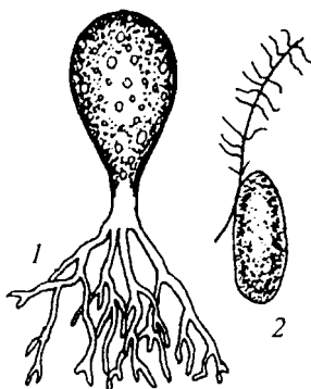
2.26-rasm. Botrydium :
