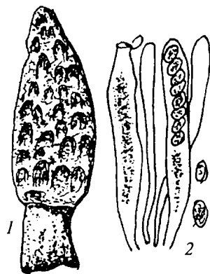
2.46-rasm. Morchella :
