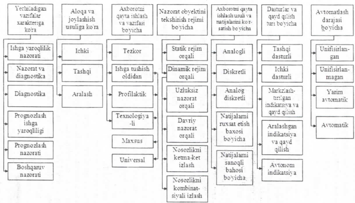
3.5 – rasm. Ichki va tashqi nazorat usullarining klassifikatsiyasi
