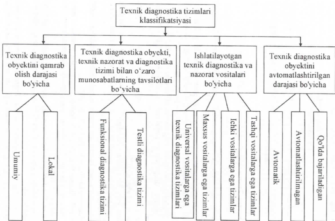
3.4-rasm. Texnik diagnostika tizimlari klassifikatsiyasining tuzilishi
