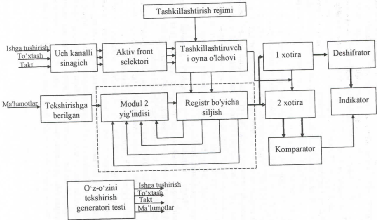
4.37-rasm. Bir kanalli SAning strukturaviy sxemasi
