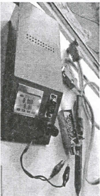
4.24- rasm. AVR markali 4-kanalli mantiqiy analizatorning umumiy ko'rinishi
