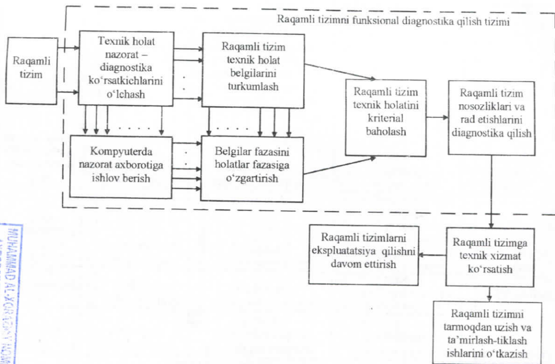
1.5 - rasm. Raqamli tizimni funksional diagnostika qilish tizimi algoritmi
