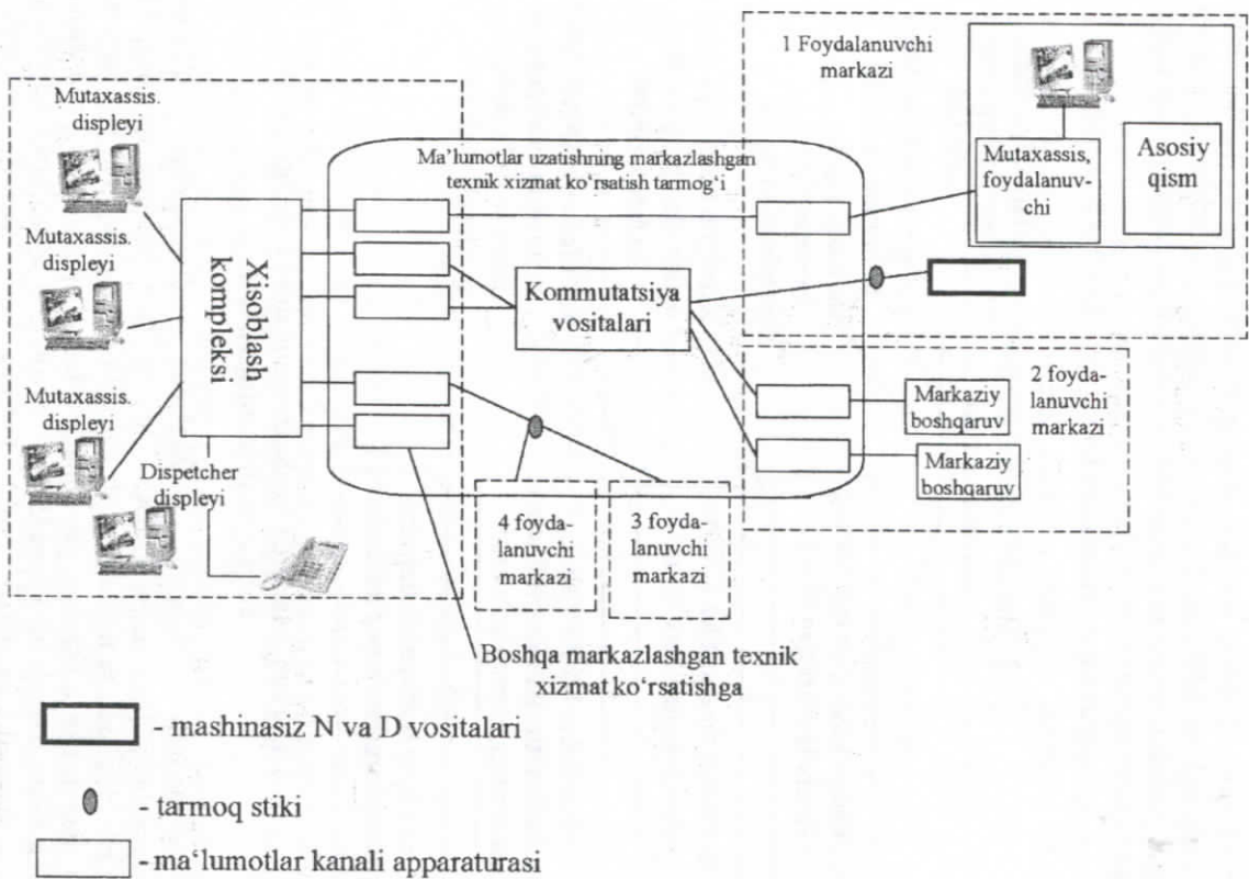
5.5-rasm. Texnik vositalar tizimining tuzilishi.
