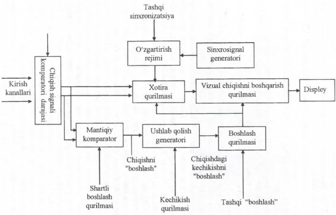
4.25-rasm. Mantiqiy analizatorning strukturaviy sxemasi
