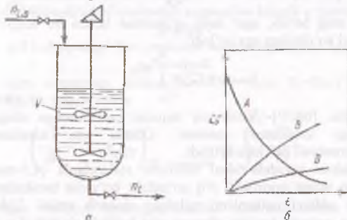
4.4-Rasm. Davriy ravishda ishlovchi ideal reaktorlar sxemasi va kiyetik o'zgarishlar grafigi.
