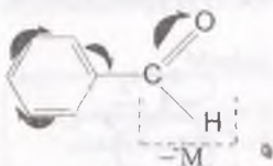
benzaldegid
