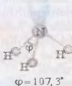
1.1-Rasm. Kimyoviy birikmalarda valent burchaklari
