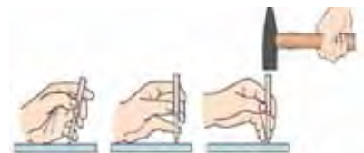
64-rasm. Plita ustida kesishda zubiloni ushlab usullari.
