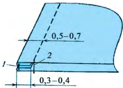
32-rasm. Qoʻsh chok.
