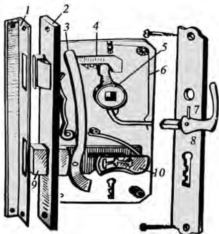
83-rasm. O‘yma qulfnig tuzilishi.
