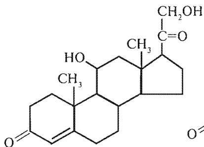
Gidrokortizon
