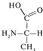
L-alanin
