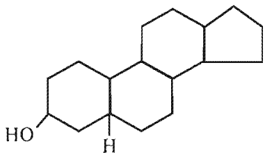
Pregnan
