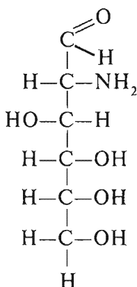
Glukozamin
