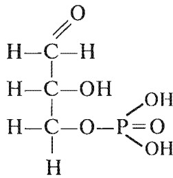
Fosfoglitserin aldegidi
