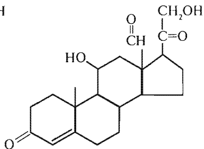
Aldosteron
