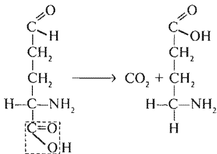
glutamin kislota
