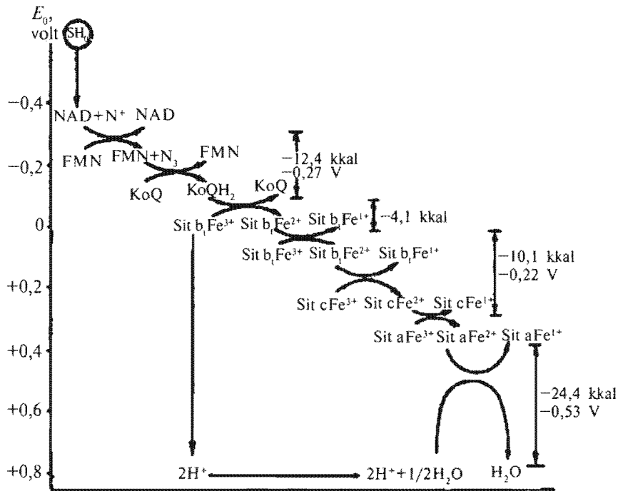
11-rasm. Elektronlarni olib o'tuvchilarning ketma-ket joylashishi.
