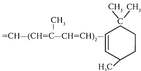
β-karotin
