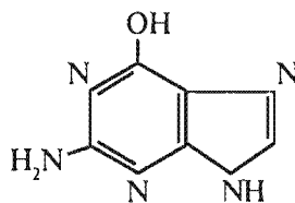
guanin
