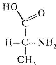
D-alanin
