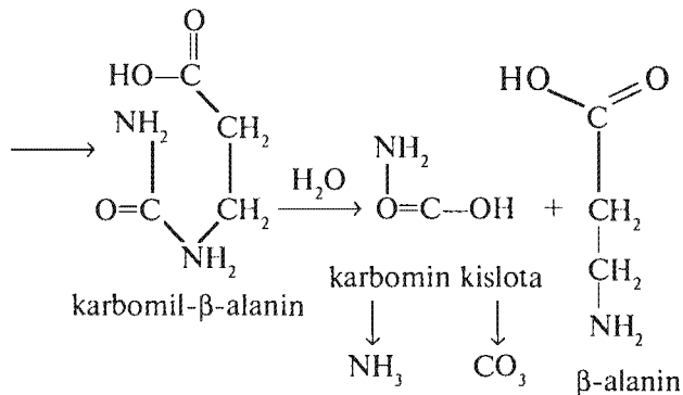
sitozin
