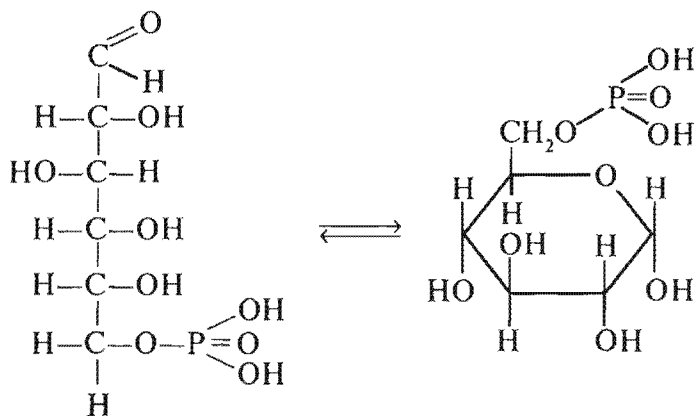
Glukoza-6-fošfat
