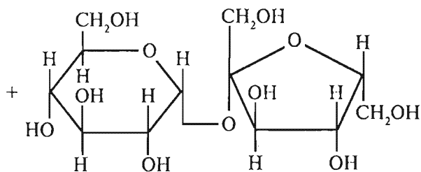
Saxaroza
