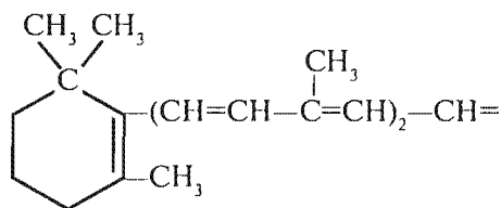
β-karotin
