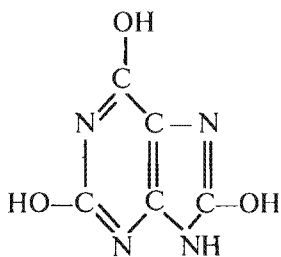
siydik kisloata
