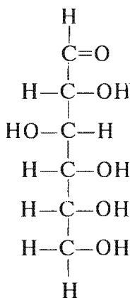
Glukoza
