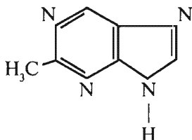
2-metiladenin
