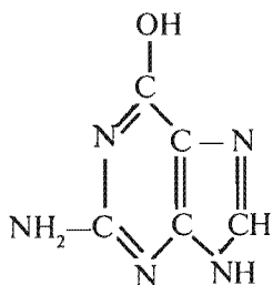
guanin
