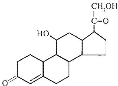
Kortikosteron
