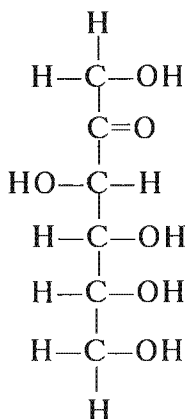
Fruktoza
