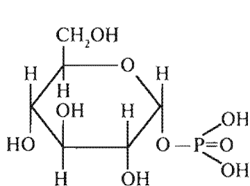
Glukoza-1-fošfat
