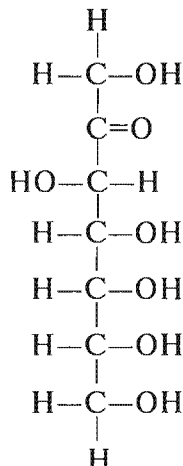
Sedogeptuloza
