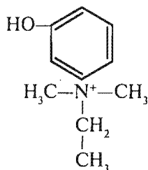
Endofoniy
