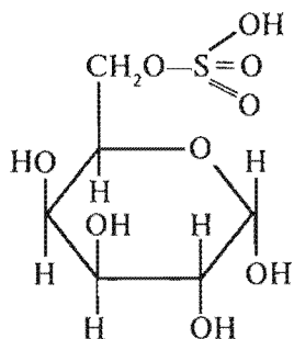
Galaktoza-6-sulfat
