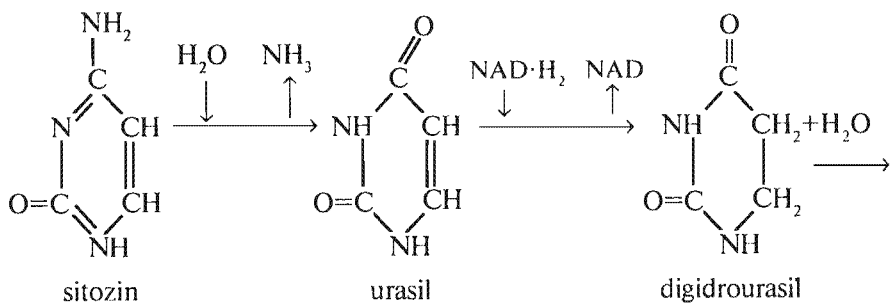
sitozin
