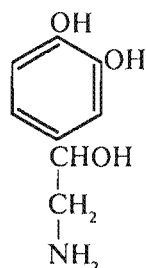
Noradrenalin
