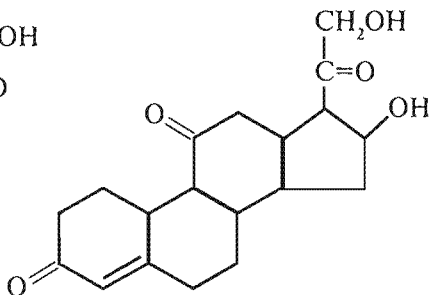
Kortizon
