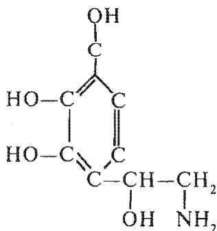
Noradrenalin
