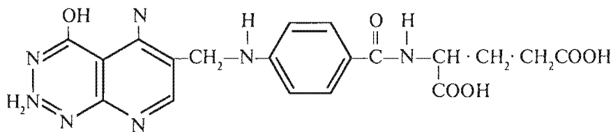
pterildin
