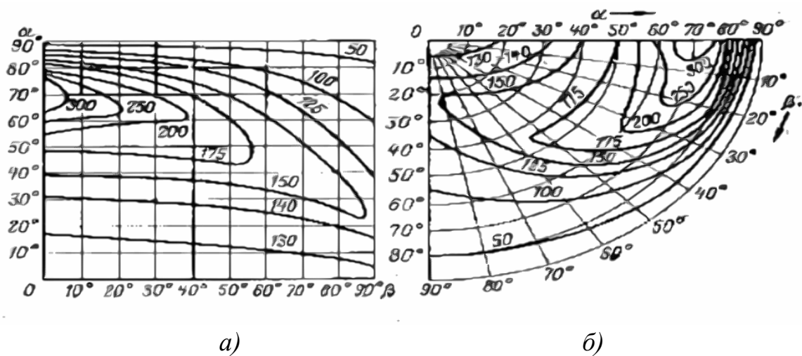
Рис. П5.2. Графики КСС несимметричных источников света
