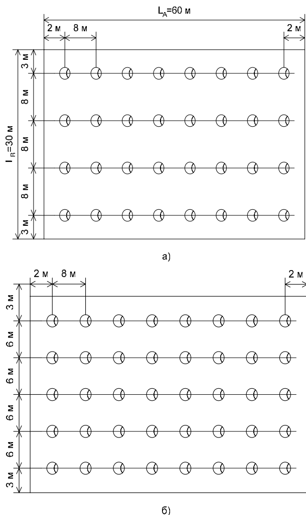
Рис. 3. Схема расположения светильников примера 2: а) – для квадратных световых полей; б) – для прямоугольных световых полей
