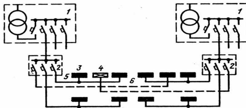
Рис. П10.2. Схема перекрестного питания рабочего и аварийного (эвакуационного) освещения производственных зданий
