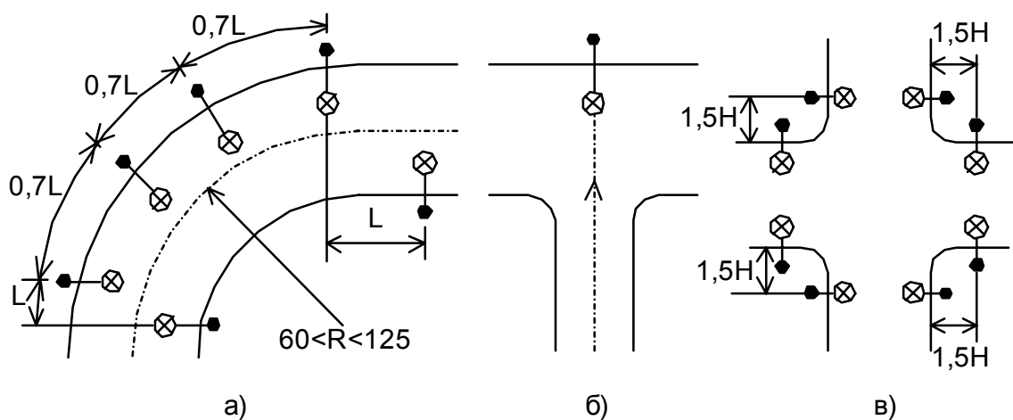
Рис. 9. Схема расположения светильников: a – на закруглении; б – на примыкании; в – на пересечении; H – высота установки светильников
