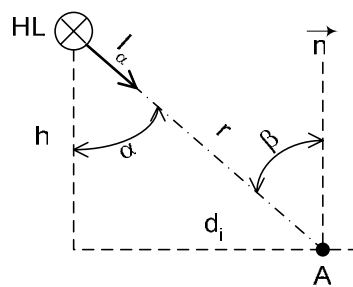
Рис. 5. К определению координат контрольной точки
