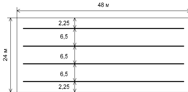
Рис. 2. Схема расположения светильников примера 1
