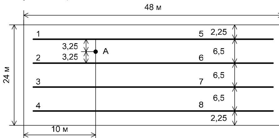
Рис. 6. Схема расположения светящихся линий примеров 3 и 7
