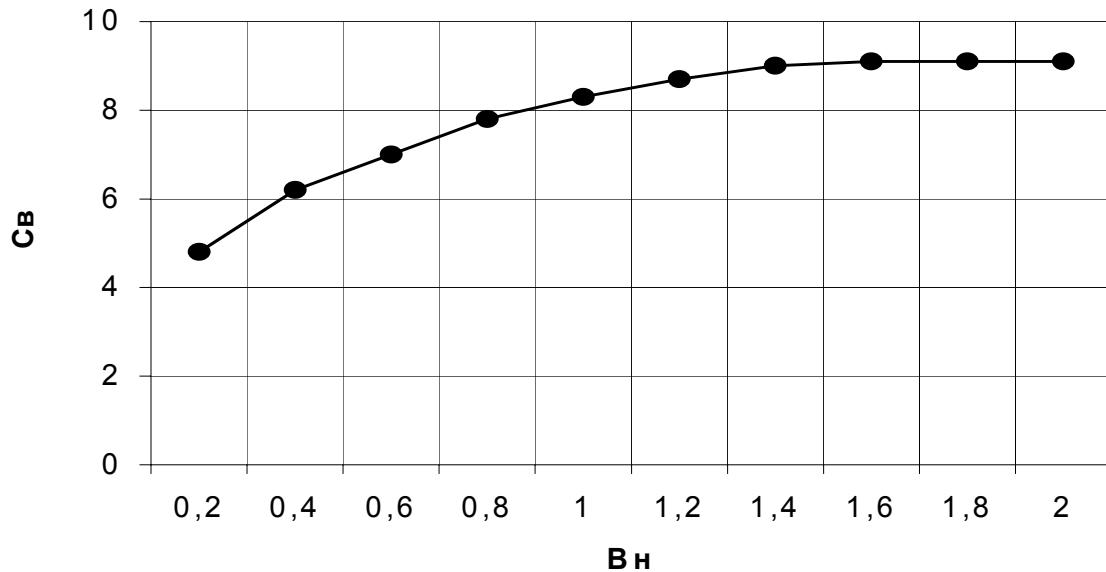
Рис. 10. График зависимости постоянного коэффициента C_B для расчета показателя ослепленности от яркости фона B_n
