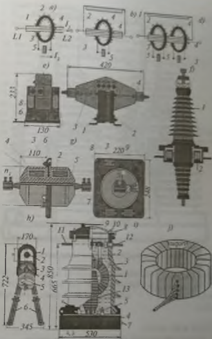
65-rasm. O'lchov tok transformatorlari:
