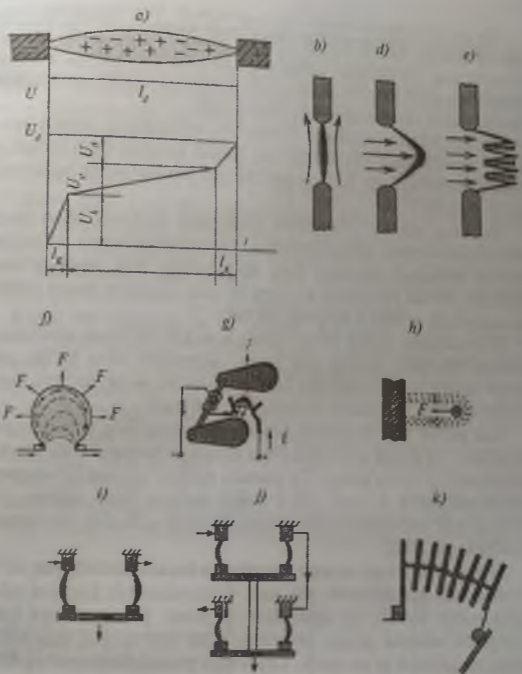
33-rasm. Elektr yoyi va yoyni so'ndirish usullari:
