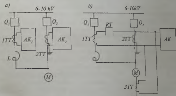
120-rasm. Reaktor bilan ishga tushiriluvchi elektr motorning ko'p fazali qisqa tutashuvdan himoyalari tok zanjirlarining sxemasi:
