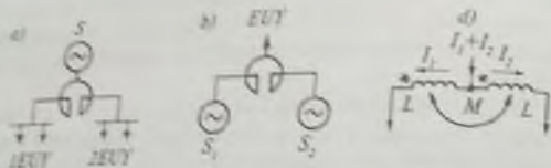
59-rasm. Reaktorlarning ulanish sxemalari:
