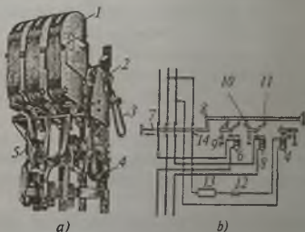
80-rasm. «A-2000» uch qutbli universal avtomat:
