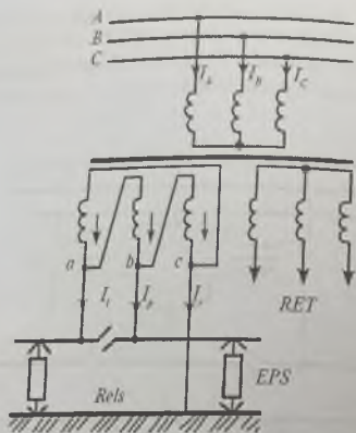
22-rasm. Kuch transformatorining ulash sxemasi: RET – hududiy elektr tarmog‘i.
