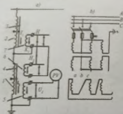
64-rasm. Kuchlanish transformatori:
