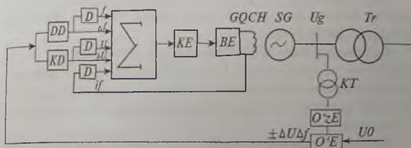
12-rasm. Kuchli ta'sir qiluvchi qo'zg'atishni avtomatik rostlagich.
