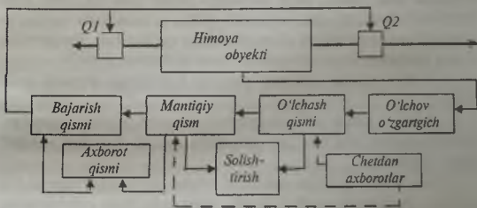
92-rasm. Releli himoya tuzilish sxemasi.
