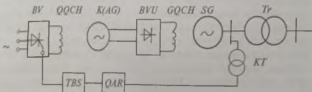
7-rasm. Katta quvvatli generatorlarda cho'tkasiz qo'zg'atish tizimlari:
