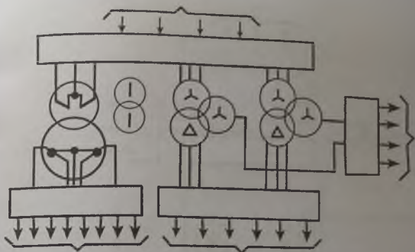
17-rasm. Uch transformatorli podstansiya.
