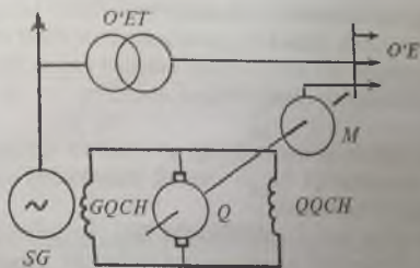
8-rasm. Generatorlarning quzg'atish tizimi:
