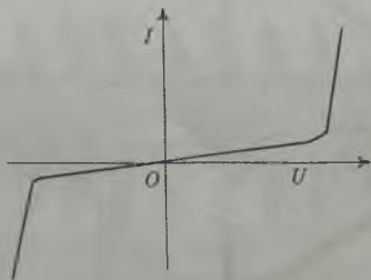
140-rasm. Ventilli razryadniklarning volt-amper tavsifi.
