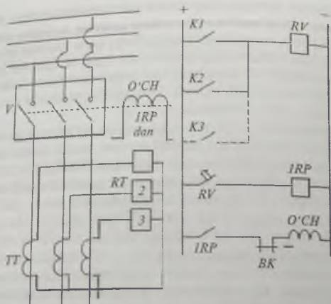
98- rasm . Maksimal tokli himoya sxema.
