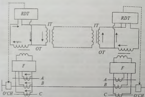
101-rasm. Bir tizimli differensial himoya.
