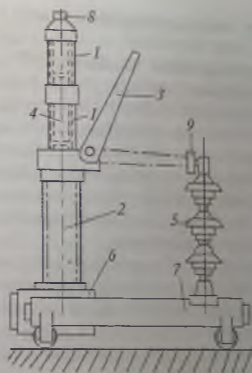
41-rasm. 110 kV kuchlanishga mo'jallangan ajratkichli havo uzgichining umumiy ko'rinishi.
