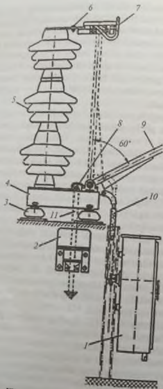
52-rasm. «KT-110» qisqa tutashtirgichining umumiy koʻrinishi: 1 – yuritma; 2 – tok transformatori; 3 – izolatori; 4 – asos; 5 – izolatorlar ustuni; 6 va 8 – qismalar; 7 – yuqori kontakt; 9 – pichoq; 10 – izolatsiyalovchi element; 11 – yerga ulovchi shina.
