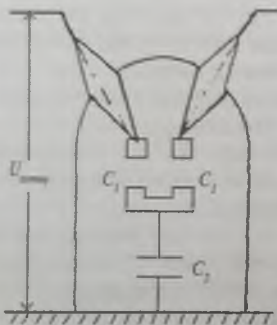
36-rasm. Yoini har bir fazada qismlarga ajratish.
