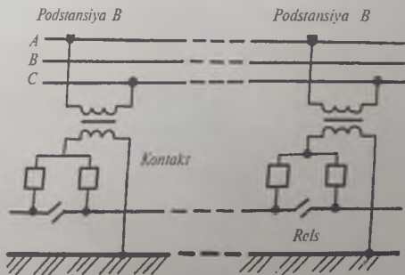
20-rasm. Bir fazali transformatorlarni ulash.
