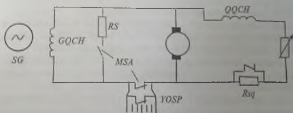
10-rasmi. Rotor chulg'ami zanjiriga tez ishlovchi avtomatning yoy so'ndiruvchi panjara YOSP ni ulash sxemasi.
