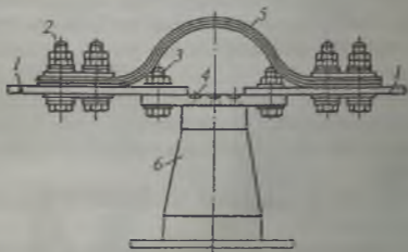
74-rasm. Shina kompensatori:
