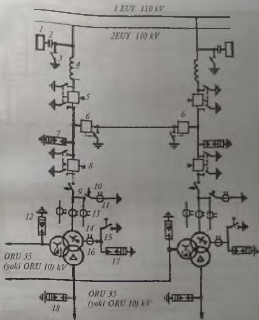
39-rasm. Podstansiya ochiq taqsimlash qurilmasi – ORU 110 kV sxemasi:
