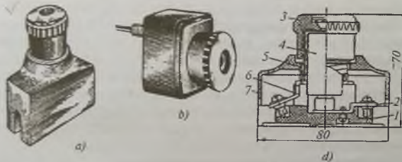
77-rasm. Bir qutbli va rezbalı saqlagichlar:
