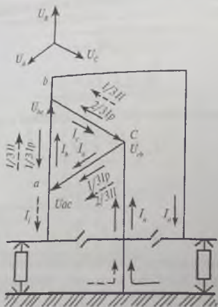
23-rasm. Kuch transformatorining ikkilamchi chulg'amlaridagi toklarning fazalar bo'yicha taqsimoti, yo'nalishi va qiymatlari.
