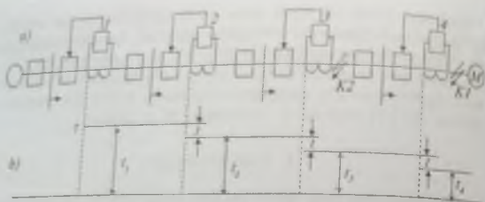
97-rasm. Bir tomonlama ta'minlanuvchi radial elektr uzatish yo'lidagi maksimal tokli himoya: a – himoyalarning joylanishi; b – pog'ona asosida joylangan himoyalarning vaqtlari.
