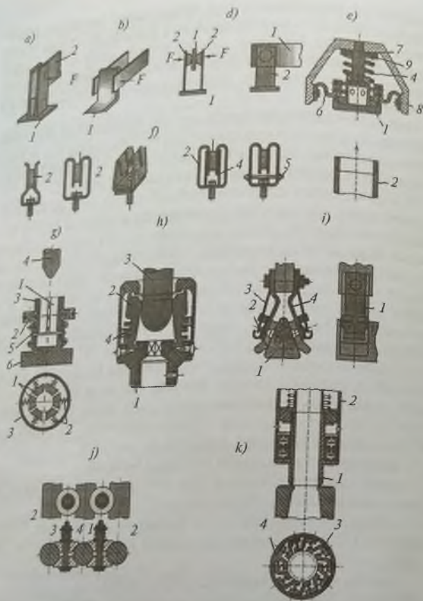
82-rasm. Operativ jihozlarning kontaktlari:
