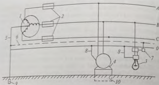
37-rasm. 380/220 V li tarmoqda elektr motor korpusi va chiroq armaturasini yerlash:
