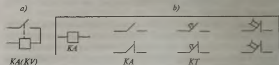
93-rasm. Relelarning tamoyil chizmalardagi shartli tasvirlari.
