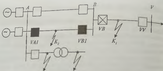
91-rasm. Shikastlangan qismlarning tanlab o'chirilishi.
