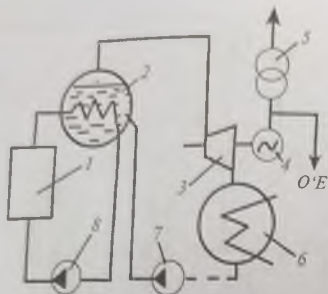
4-rasm. Atom-elektr stansiyasining sxemasi:
