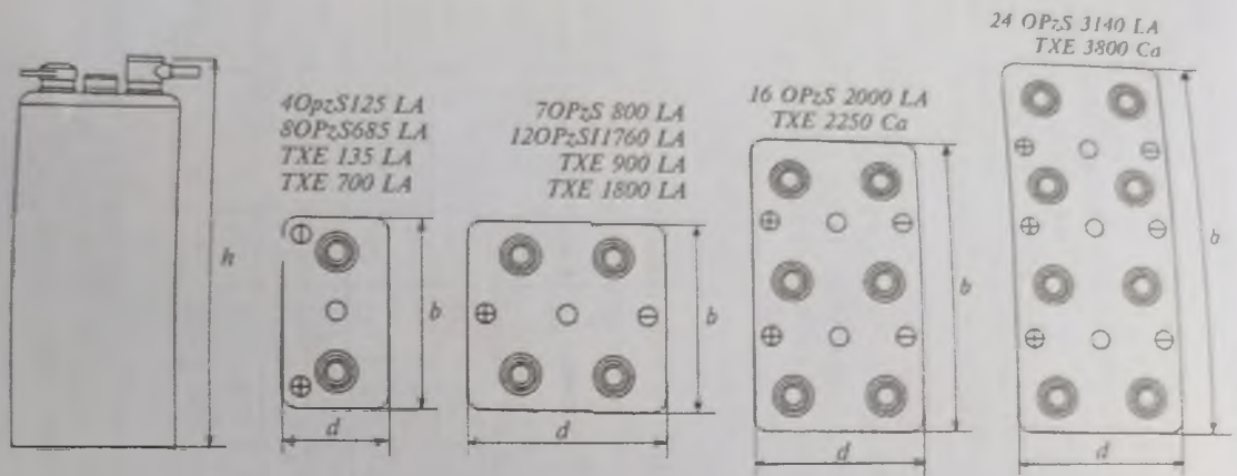
124-rasm. OPzV va TXE rusmli qo'rg'oshin-kislotali akkumulatorning tashqi o'lchamlari.
