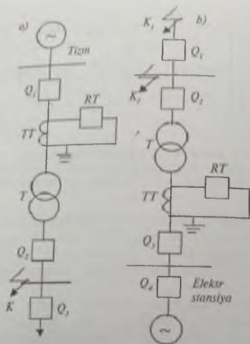
106-rasm. Transformatorlarni katta tokdan himoya sxemasi: a – pasaytiruvchi transformatorlar uchun; b – kuchaytiruvchi transformatorlar uchun.
