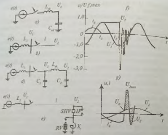
86-rasm. Elektr uzatish yo'lining ulanish usullari:
