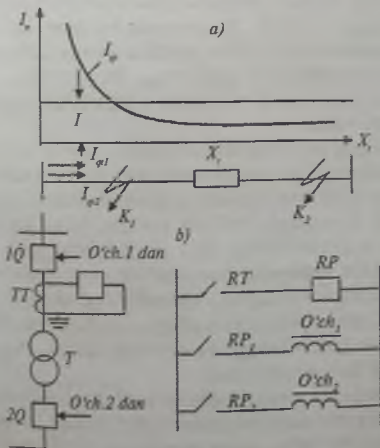
113-rasm. Transformatorning tokli kesim himoyasi: a - ishlashi asosi; b - bir chiziqli sxemasi.
