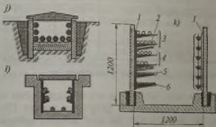
75-rasm. Yuqori kuchlanishli kabel kesimi va yotqizish usullari:
