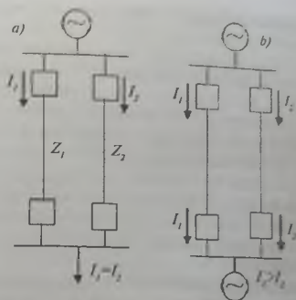
102-rasm. Parallel elektr uzatish yo'llari ko'ndalang differensial himoyasi: a — me'yorli-normal yukdagi toklar; b — bir uzatish yo'lidagi qisqa tutashuvdagi toklar ko'rsatilgan.
