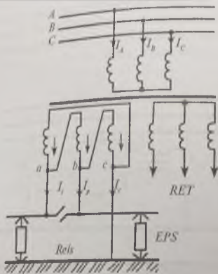
22-rasm. Kuch transformatorining ulash sxemasi: RET – hududiy elektr tarmogʻi.
