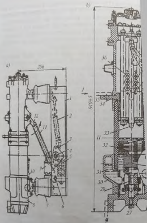
43-rasm. BMI-10K uzgichi: a – ulangan va b – uzilgan holati.
