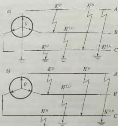
88-rasm. Qisqa tutashuvning turlari.
