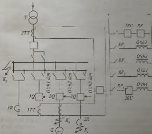
118-rasm. Reaktorli va bir necha manbasi bo'lgan taqsimlash punktlarining to'liq bo'lmagan differensial himoya sxemasi.
