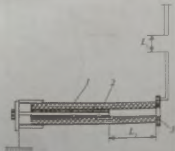
138-rasm Quvurli razryadniklar:
