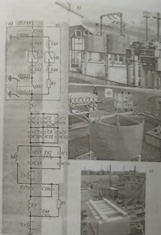
131- rasm. Filtrlash va kompensatsiyalash qurilmasi
