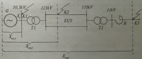
89-rasm. Qisqa tutashuv joyini belgilovchi sxema.
