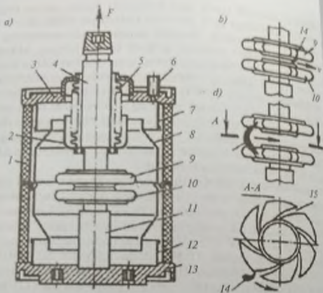
47-rasm. BBΦ-27,5 vakuumli uzgich kamerasi ning tuzilishi:
