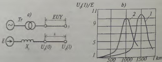
85-rasm. Tok manbayi – generator E, transformator Tr va elektr uzatish yo'llaridan tuzilgan simmetrik uch fazali holatda kuchlanishning kattalashib ketishi:
