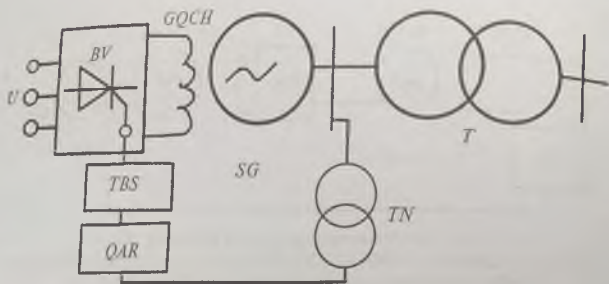
6-rasm. Katta quvvatli generatorning yuqori chastotali qo'zg'atish tizimi:
