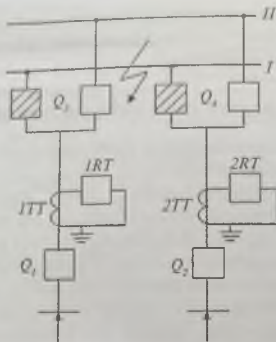
117-rasm. Ikki uzgichli pasaytiruvchi stansiya himoyasi.
