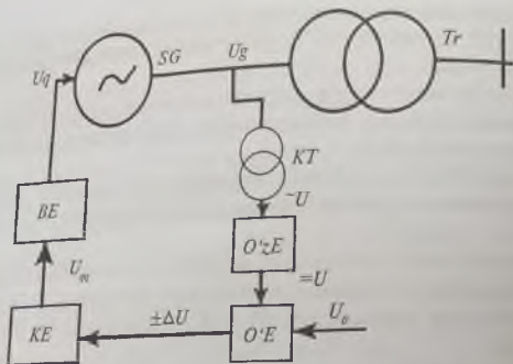
11-rasm. Kuchli ta'sir qiluvchi qo'zg'atishni avtomatik rostlagich: O'zE – o'zgartiruvchi element; O'E – o'lchov elementi; KE – kuchaytiruvchi element; BE – bajaruvchi element.
