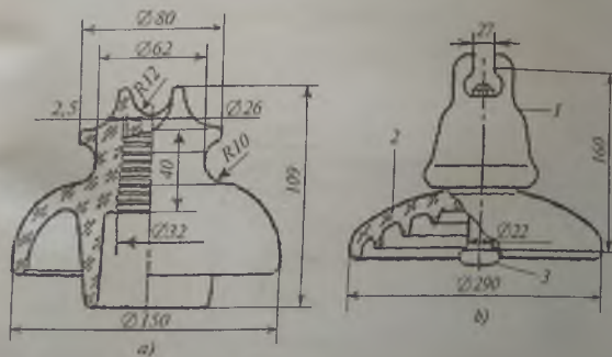
69-rasm. Izolatorlarning tashqi ko'rinishi:
