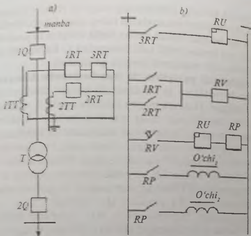
107-rasm. Bir tomonlama ta'minlanuvchi bunday transformatorning sxemasi:
