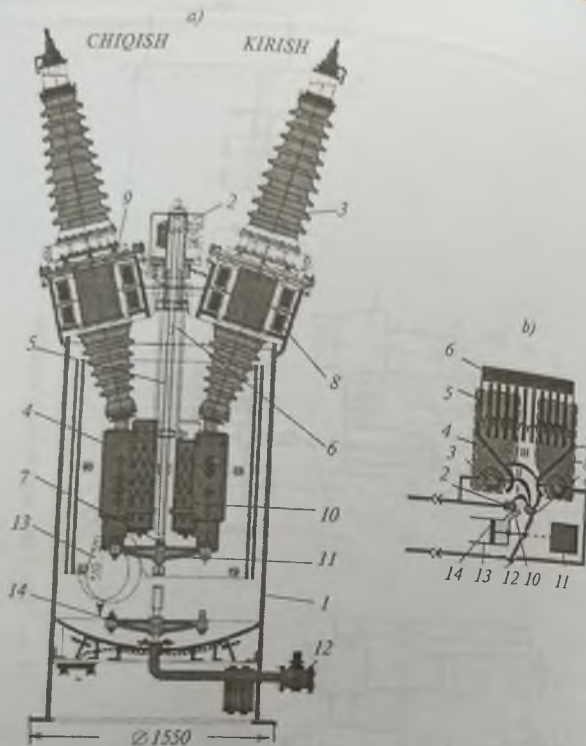
45-rasm. Moyli (a) va elektromagnit (b) uzgichlar:
