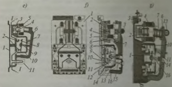
81-rasm. Kontaktorlar va magnit yurtkichlar:
