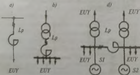
54-rasm. Reaktorlarning ulanish sxemalari:
