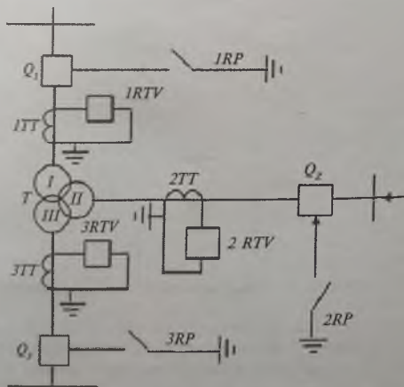
109-rasm. Transformatorlarning tashqi qisqa tutashuvlarga ta'sir sxemasi.
