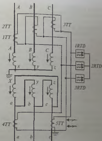
115-rasm. Transformatorning differensial tokli kesim himoyasi.
