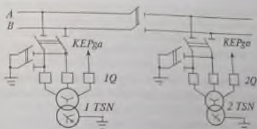
123-rasm. Podstansiyalarning o'z ehtiyoj transformatorlarini ulash sxemalari.
