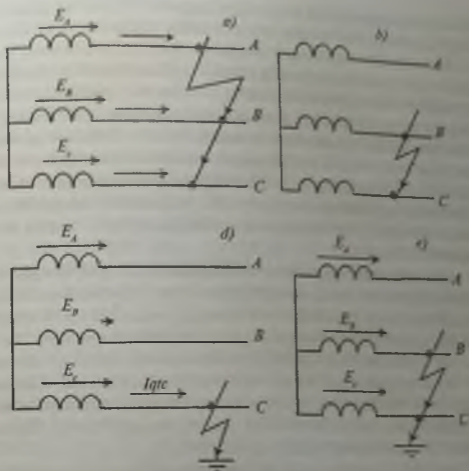
83-rasm. Qisqa tutashuvlarning turlari:
