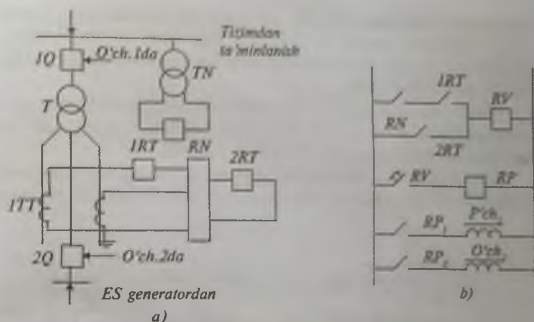
110-rasm. Transformatorlarning tashqi qisqa tutashuvlarga ta'sir sxemasi.
