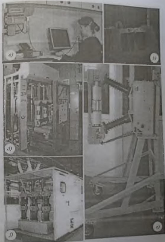
134- rasm. Taqsimlovchi qurilmalar.
