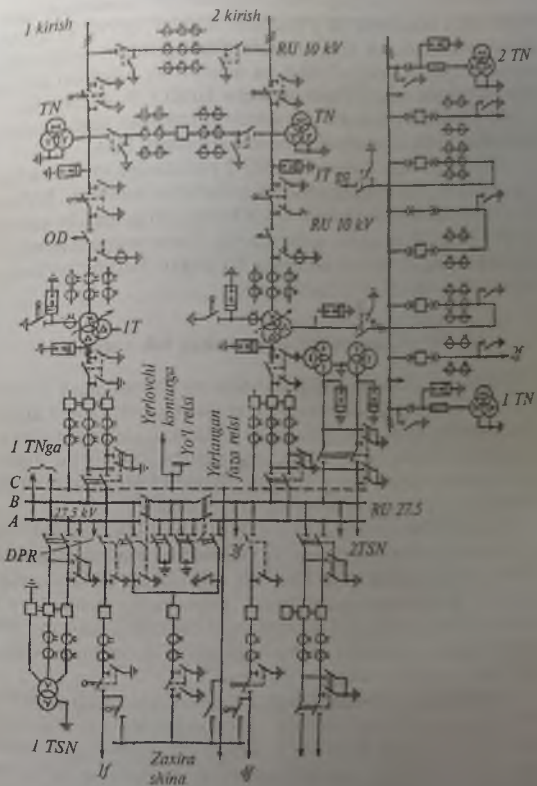
38-rasm. Podstansiyasining bosh elektr ulash sxemasi:
