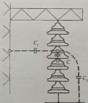
70-rasm. Izolator shodasi.
