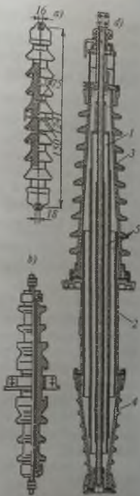
71-rasm. Izolatorlarning tashqi ko'rinishi: a - tayoqcha osma izolator; b - kirma izolator; d - kirma izolatorning qirqimi.
