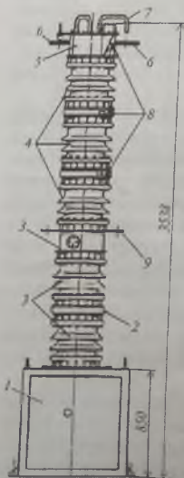
48-rasm. BBΦ-27,5 uzgichining tashqi ko'rinishi.
