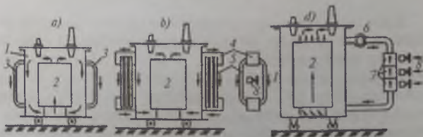
32-rasm. Kuch transformatorlarining sovitish tizimlari:
