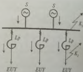
59-rasm. Qisqa tutashuv holatida reaktorning induktiv qarshiligining o'zgarishi.
