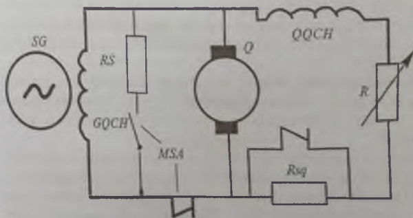
9-rasm. Rotor chulg'amini so'ndiruvchi faol qarshilikka ulash sxemasi:
