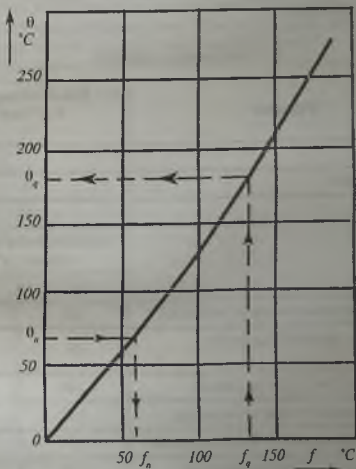
90-rasm. f ning harorat \Theta ga bog'liqlik grafigi.
