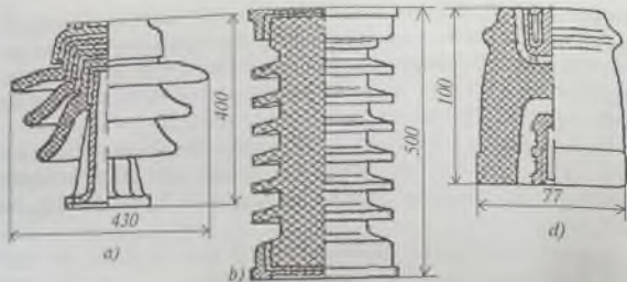
67-rasm. Izolyatorlarning tashqi ko'rinishi:
