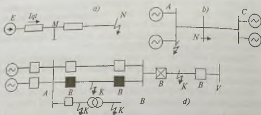
87-rasm. a – EUY oxirida sodir bo'lgan qisqa tutashuv; b – «A» elektrostansiyasiga yaqin joyda sodir bo'lgan qisqa tutashuv; d – sxemadagi shikastlangan qismlarni selektiv o'chirishi.
