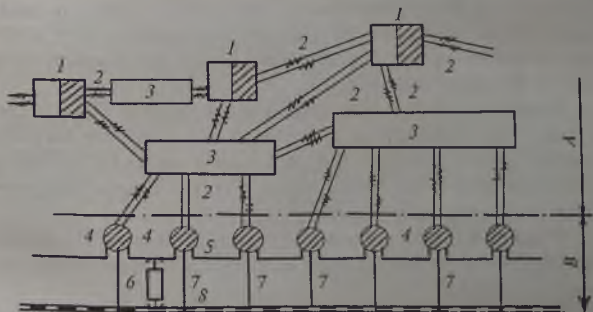
13-rasm. Yuklamalarini elektr bilan ta'minlash sxemasi:
