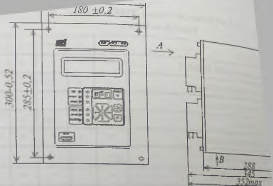
121-rasm. BMRS bloklarning tashqi ko'rinishi.
