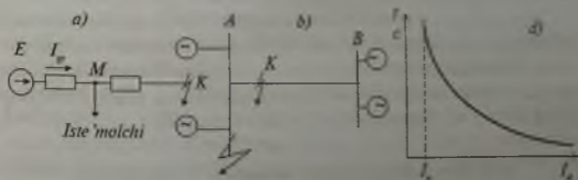
84-rasm. Qisqa tutashuvning kuchlanish tushishiga ta'siri:
