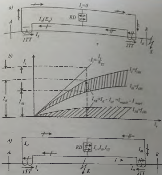
99-rasm. Differensial himoyaning ishlashi: a – tashqi qisqa tutashuvda; b – nobalanslik toklari; d – himoyalananayotgan yo‘lda qisqa tutashuvda.
