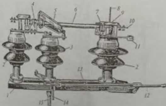
51-rasm. «RLNZ-35/600» ajratkichi:
