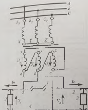
15-rasm. Yulduz-uchburchak ulanish guruhi kuch transformatorini tarmog'iga ulash sxemasi:
